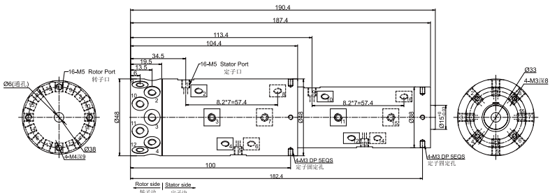
MQR16 尺寸图 16进16出, M5牙
