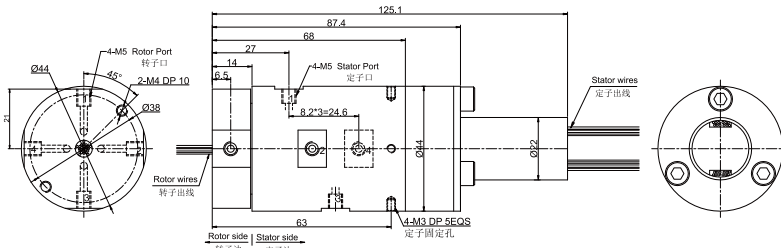
MQR4-S24 尺寸图 4进4出, M5牙 + 24路信号(2A)
