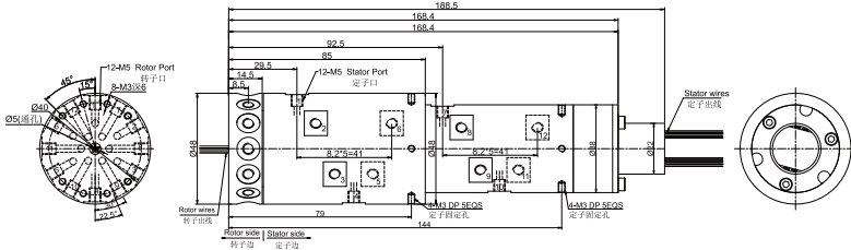
MQR12-S24 尺寸图 12进12出, M5牙 + 24路信号(2A)
