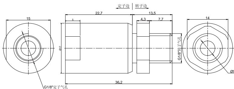
MK11A 尺寸图
