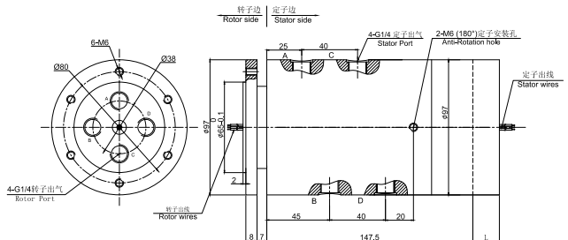
MAPH400S-03 尺寸图
