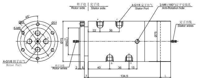
MAPH400S-03 尺寸图
