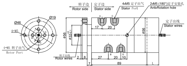
MAPH400S-02 尺寸图
