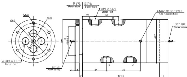
MAPH400S-05 尺寸图
